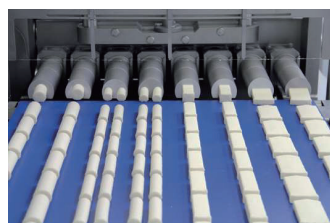
FS 510 による多彩な成形形状例
