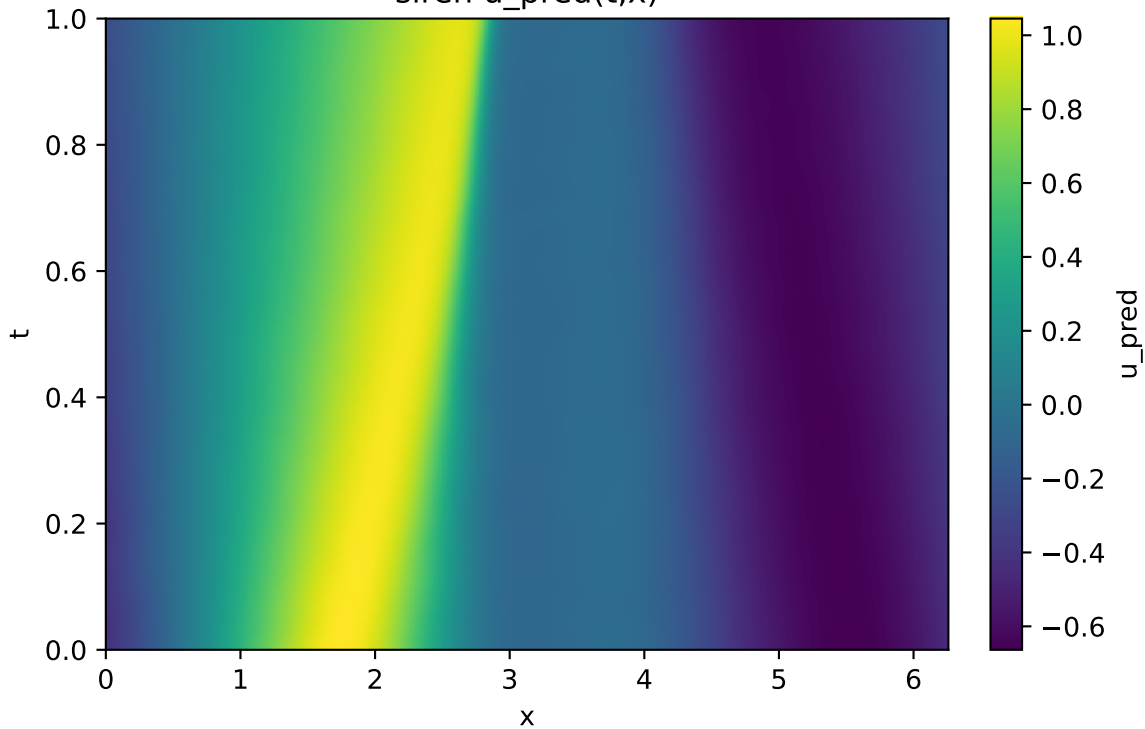
siren u_{\text{pred}}(t,x)
