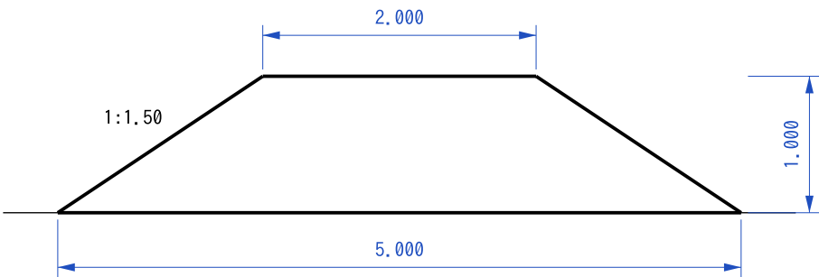
側 面 図
