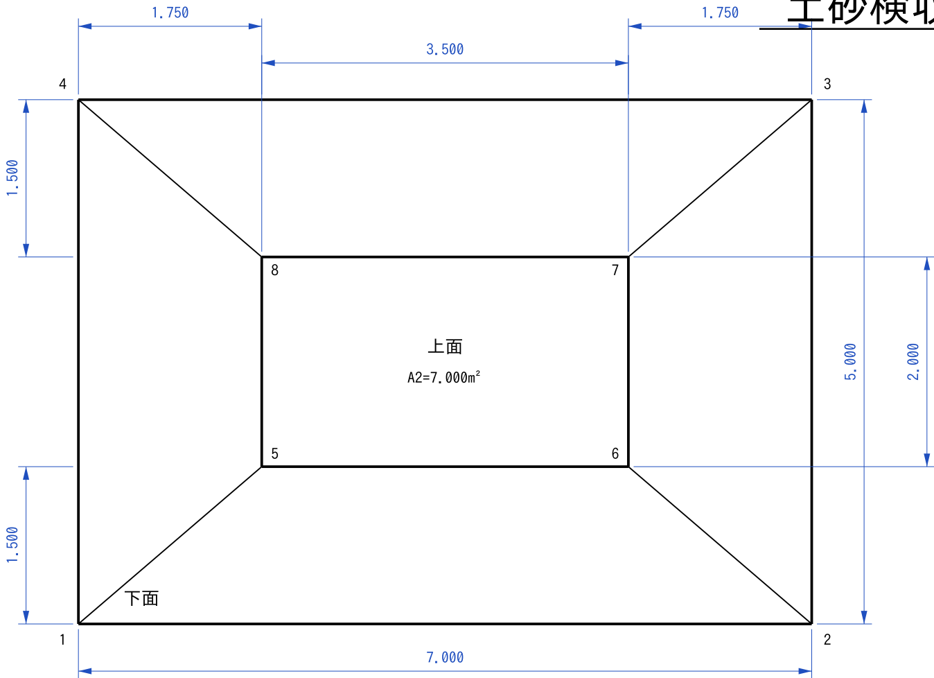
平 面 図
