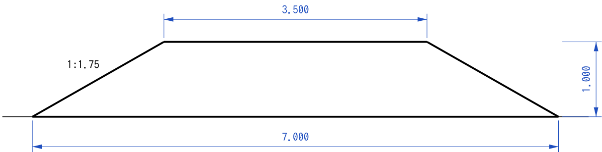
正 面 図
