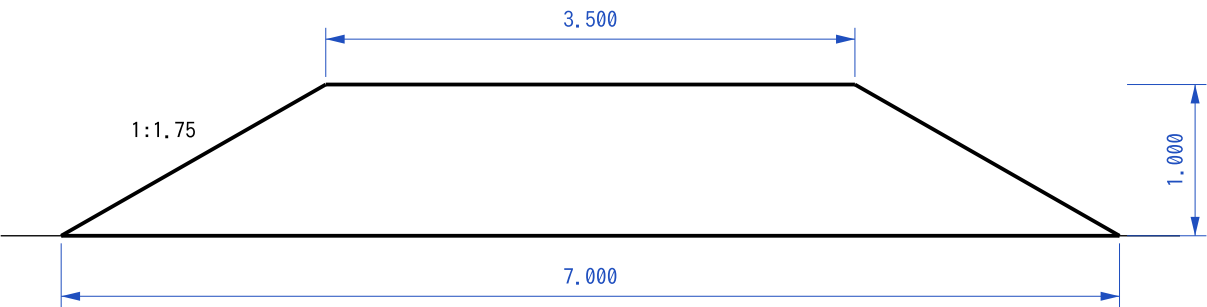
正 面 図
