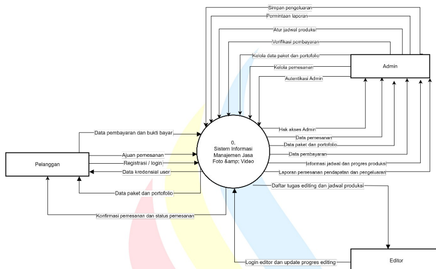
Gambar BAB IV HASIL DAN PEMBAHASAN.4 Diagram Konteks
