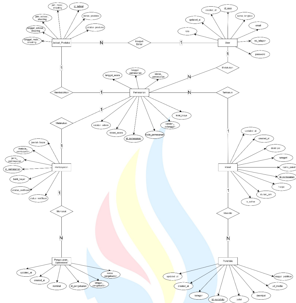
Gambar BAB IV HASIL DAN PEMBAHASAN.13 Entity Relationship Diagram
