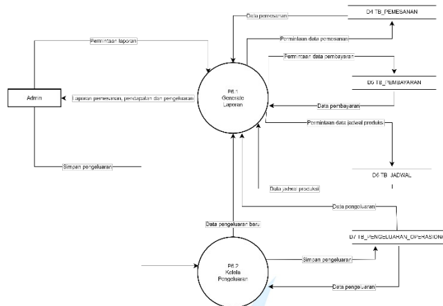
Gambar BAB IV HASIL DAN PEMBAHASAN.11 DFD Level 1 - Proses 6 (Pelaporan)
