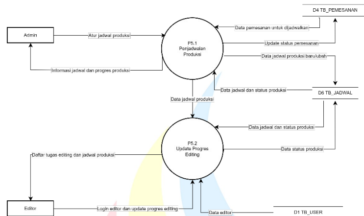
Gambar BAB IV HASIL DAN PEMBAHASAN.10 DFD Level 1 - Proses 5 (Penjadwalan Produksi dan Editing)
