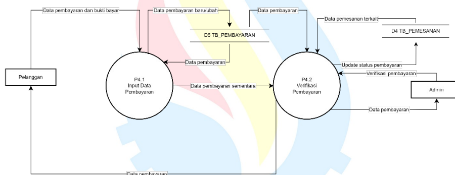
Gambar BAB IV HASIL DAN PEMBAHASAN.9 DFD Level 1 - Proses 4 (Kelola Pembayaran)
