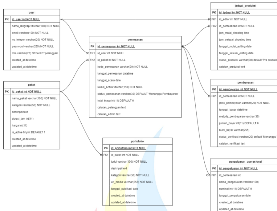
Gambar BAB IV HASIL DAN PEMBAHASAN.12 Konseptual Basis Data
