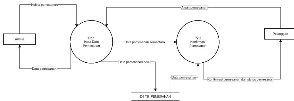
Gambar BAB IV HASIL DAN PEMBAHASAN.7 DFD Level 1 - Proses 2 (Kelola Pemesanan)
