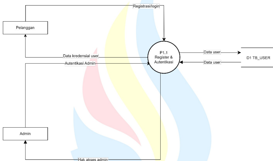
Gambar BAB IV HASIL DAN PEMBAHASAN.6 DFD Level 1 - Proses 1 (Autentikasi User)
