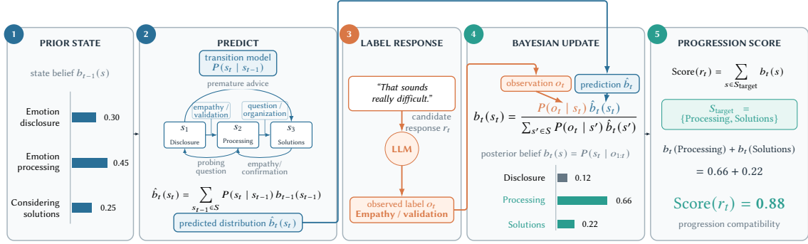
Fig. 2. Dialogue Progression Scoring Moduleにおける候補応答の評価処理の模式例。前ターンまでの状態分布を遷移モデルにより予測し、候補応答から得た観測ラベルを用いてベイズ更新を行う。青色の経路は予測分布、橙色の経路は観測ラベルが更新式のどの項へ入力されるかを示す。例では、更新後の分布における対象状態ProcessingとSolutionsの確率を合計し、Score = 0.88を得る。
