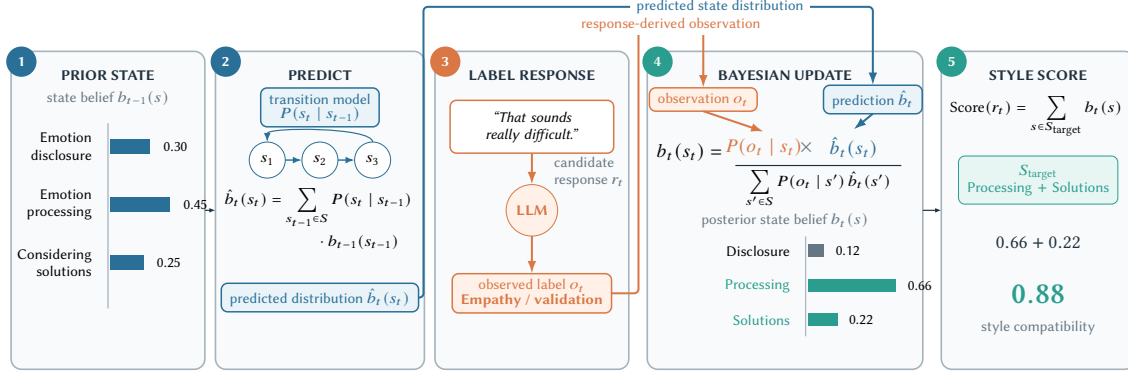
Fig. 2. Style Compatibility Scoring Moduleにおける候補応答の評価処理の模式例。前ターンまでの状態分布を遷移モデルにより予測し、候補応答から得た観測ラベルを用いてベイズ更新を行う。青色の経路は予測分布、橙色の経路は観測ラベルが更新式のどの項へ入力されるかを示す。例では、更新後の分布における対象状態ProcessingとSolutionsの確率を合計し、Score = 0.88を得る。
