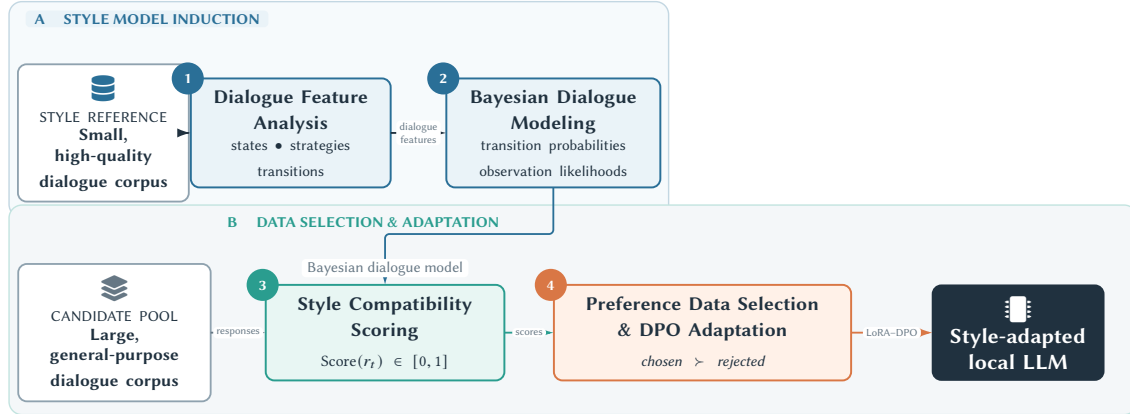
Fig. 1. BASiSの全体構成．上段では、小規模高品質コーパスから会話特徴を抽出し、ベイズ的対話モデルを構築する．下段では、構築したモデルによって大規模汎用コーパスの候補応答をスコアリングし、得られた選好データを用いたLoRA-DPOによりローカルLLMを適応させる．丸数字は本文で説明する4つのモジュールに対応する．
