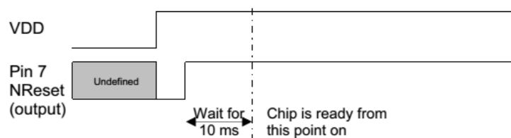
Figure 42. POR Timing Diagram
