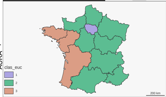
1.b CAH-REG en 3 classes
