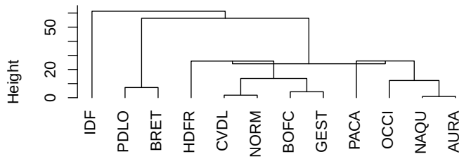
1.a Distance euclidienne non standardisée
