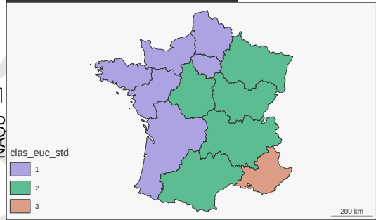
2.b CAH-REG en 3 classes
