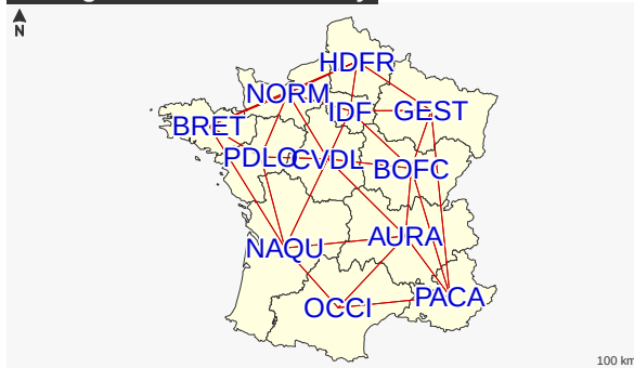
Triangulation de Delaunay
