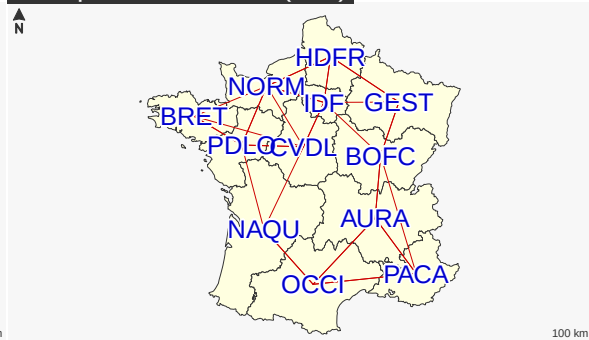
Plus proches voisins (k=3)
