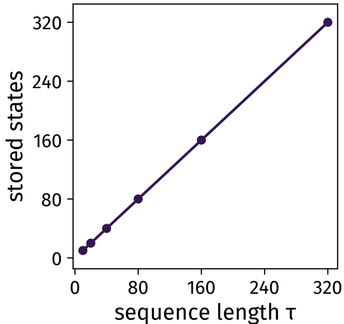
(b) memory, O(\tau)
