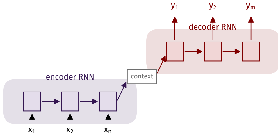
(d) encoder-decoder
