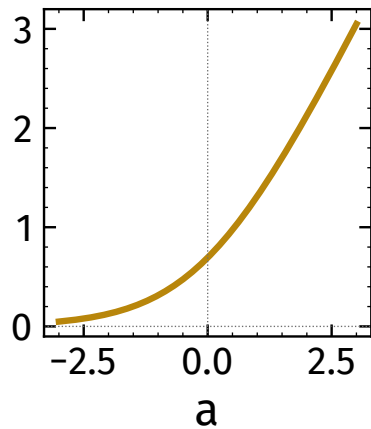
softplus \ln(1 + e^a)
