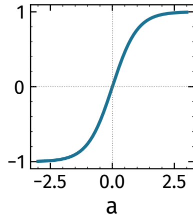
tanh \tanh a
