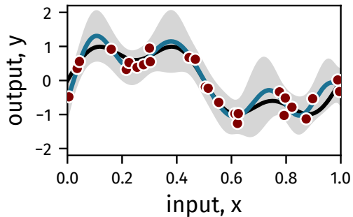
(d) predictive mean, \pm 2 s.d.
