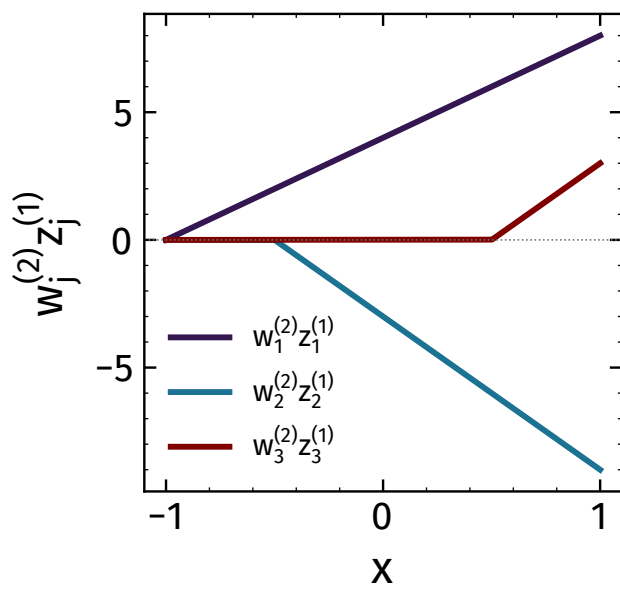
(d) weighted units of layer 1
