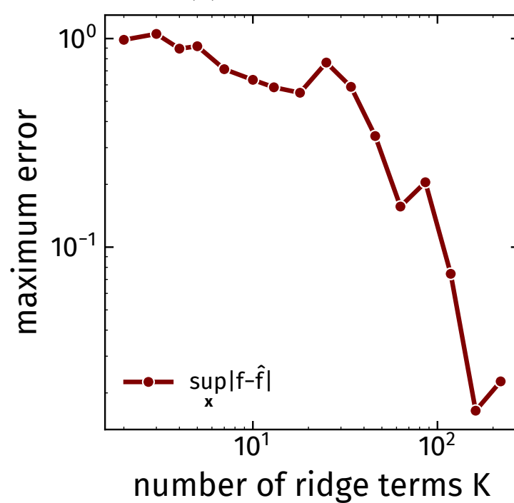
(d) error \rightarrow 0 as K \rightarrow \infty
