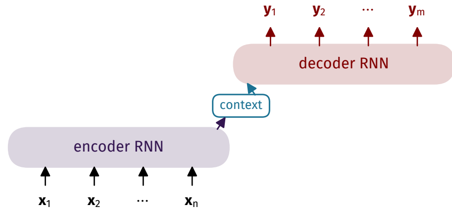
(d) encoder--decoder
