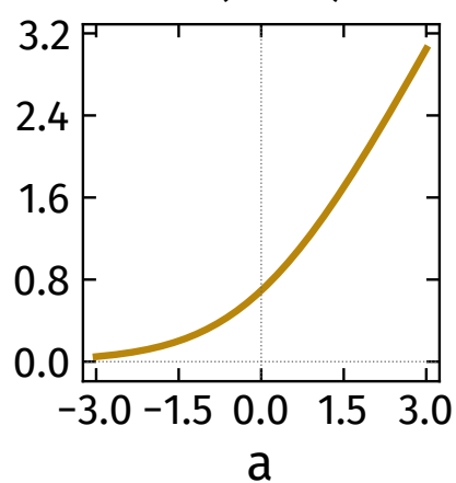
softplus \ln(1 + e^a)
