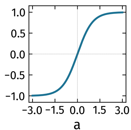
tanh \tanh a
