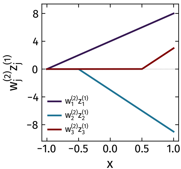
(d) weighted units of layer 1
