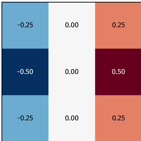
\mathbf{W}_1 : vertical edge
