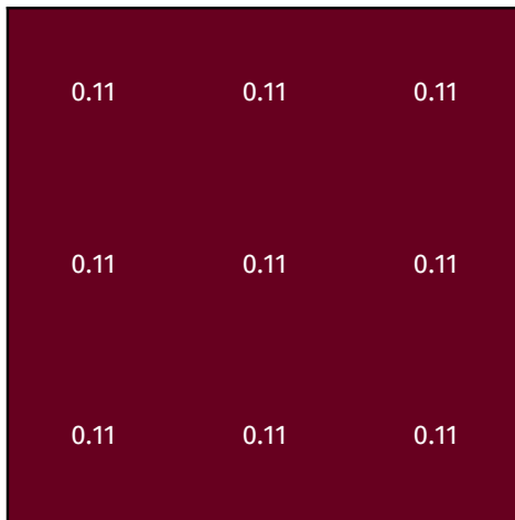
\mathbf{W}_2 : blur
