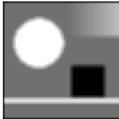
blur \alpha_3 = -0.100
