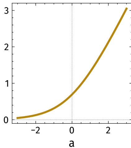
softplus \ln(1 + e^a)
