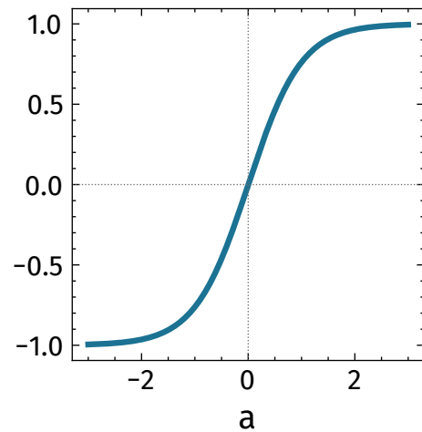
tanh \tanh a
