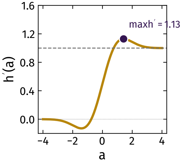
GELU
