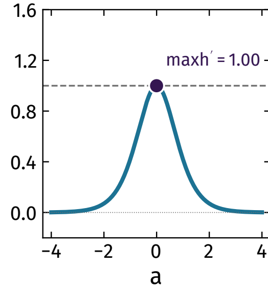
tanh
