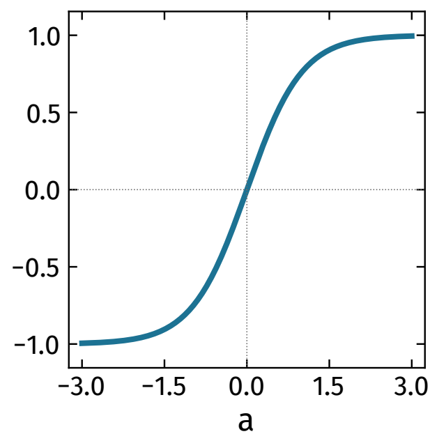
tanh \tanh a
