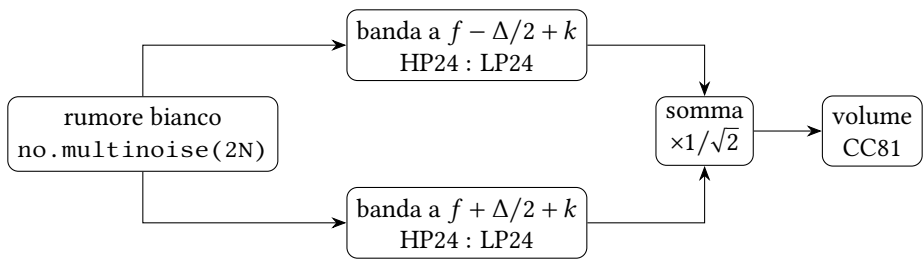
Un canale k di LMO; i quattro canali sono uguali, con flussi di rumore diversi.
