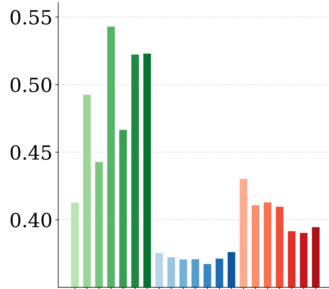
LPIPS ↓
