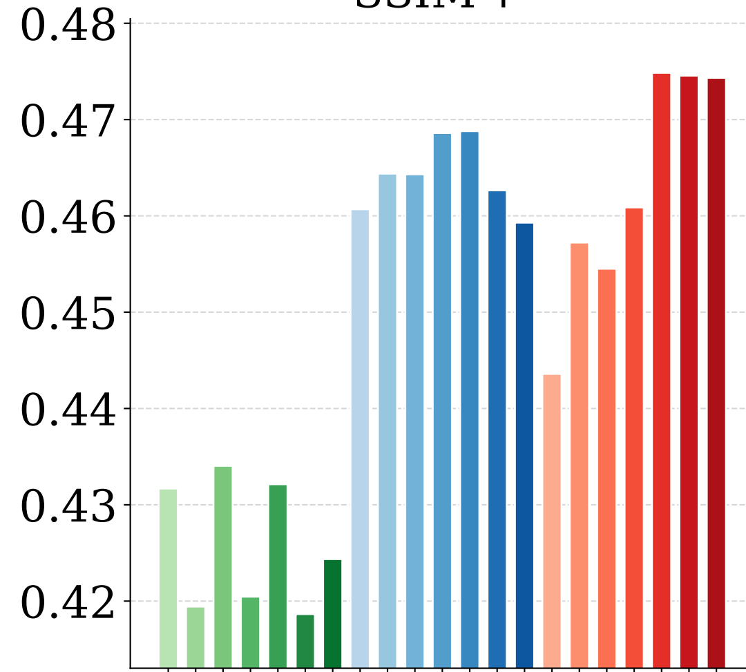
SSIM ↑
