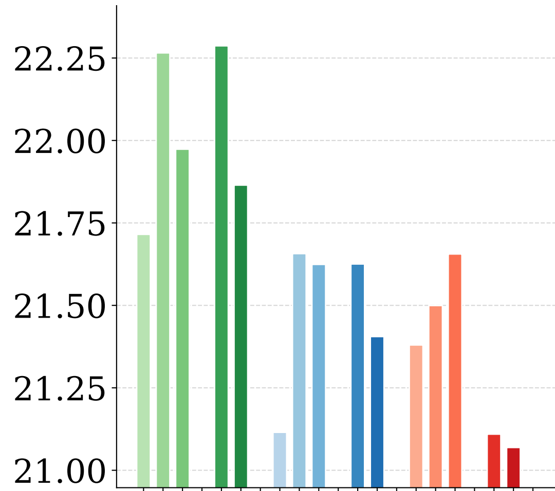
PSNR \uparrow
