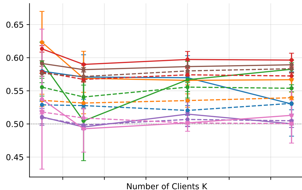
TPR @ FPR ≤ 0.01
