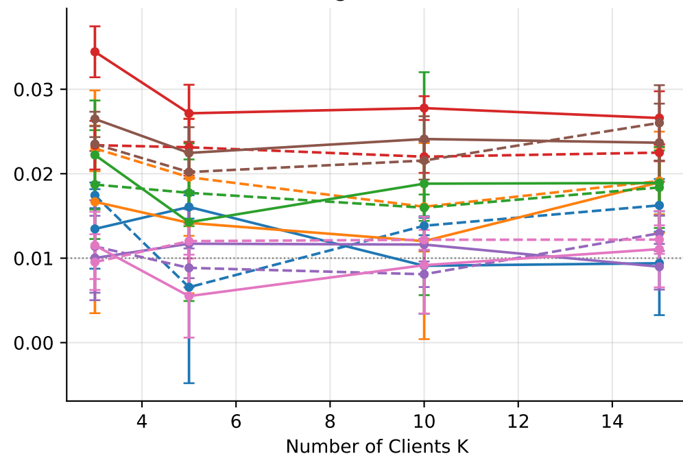
TPR @ FPR ≤ 0.01
