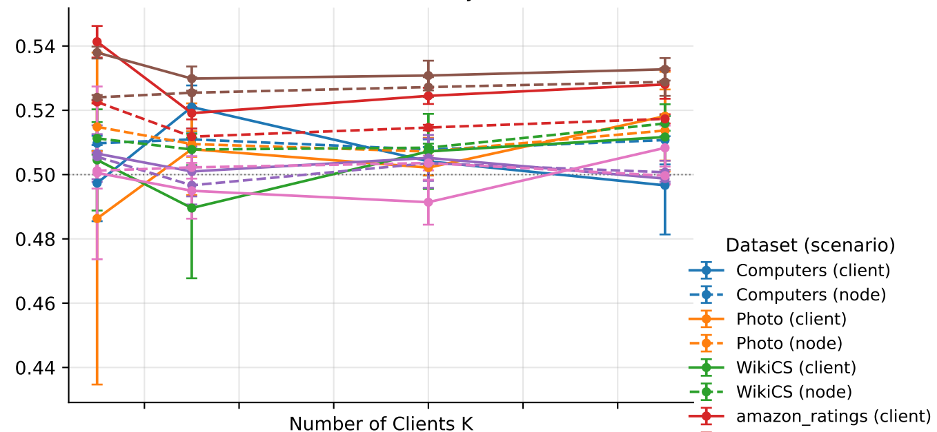
TPR @ FPR ≤ 0.001
