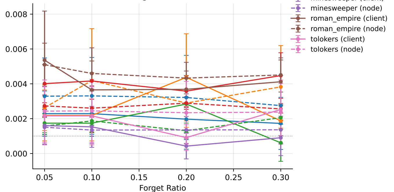
TPR @ FPR ≤ 0.001
