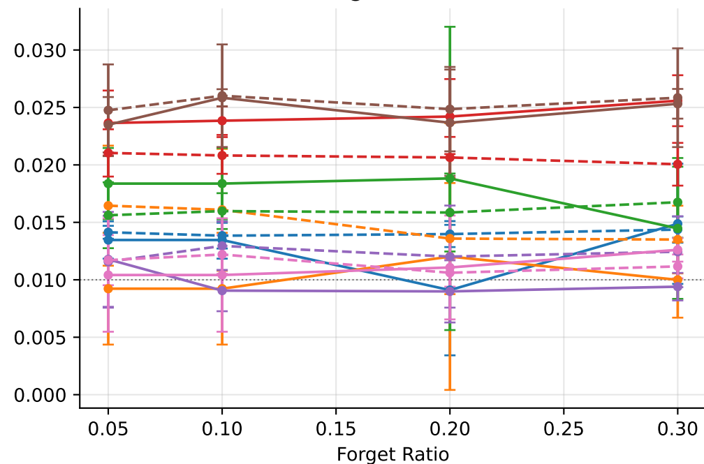
TPR @ FPR ≤ 0.01
