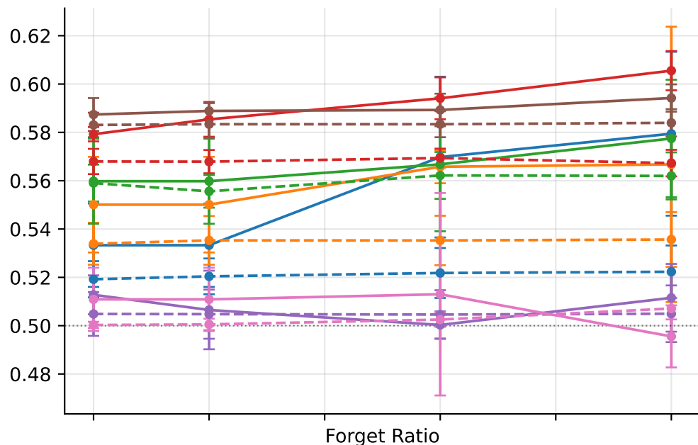
TPR @ FPR ≤ 0.01
