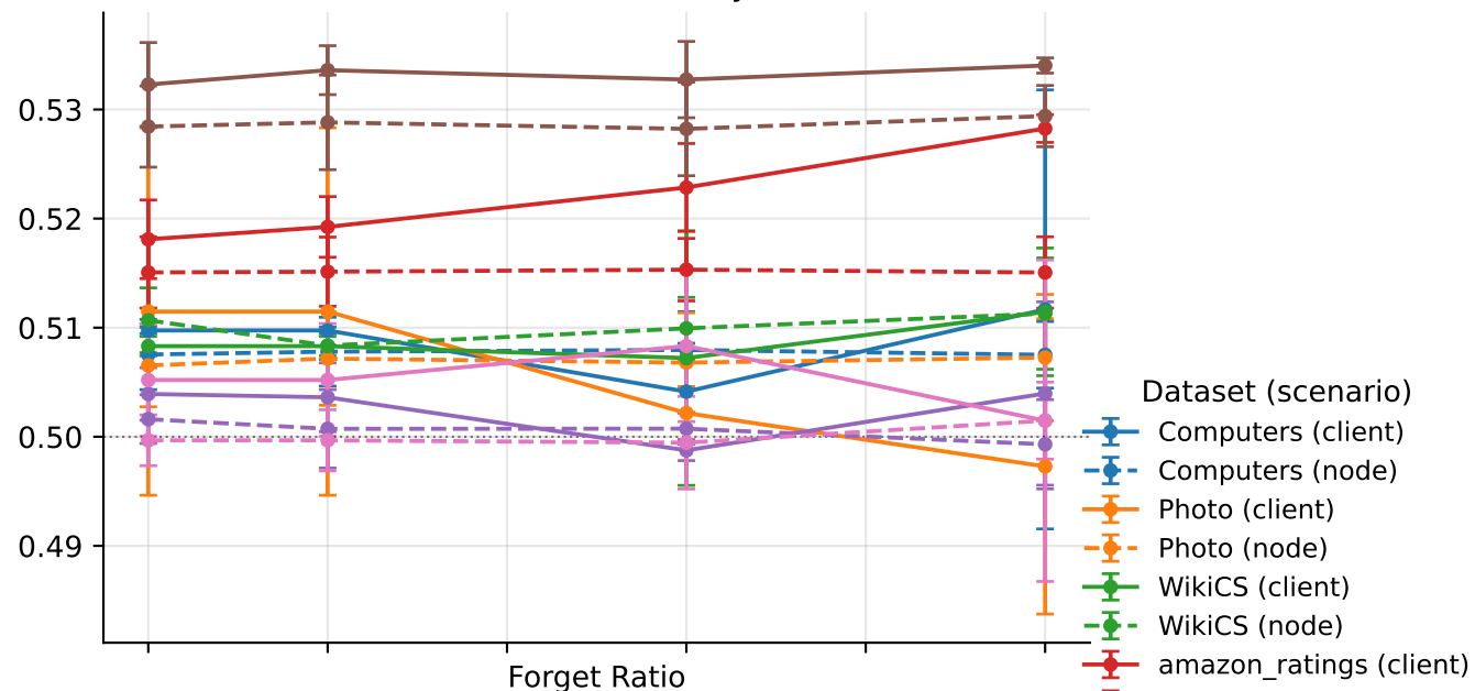
TPR @ FPR ≤ 0.001
