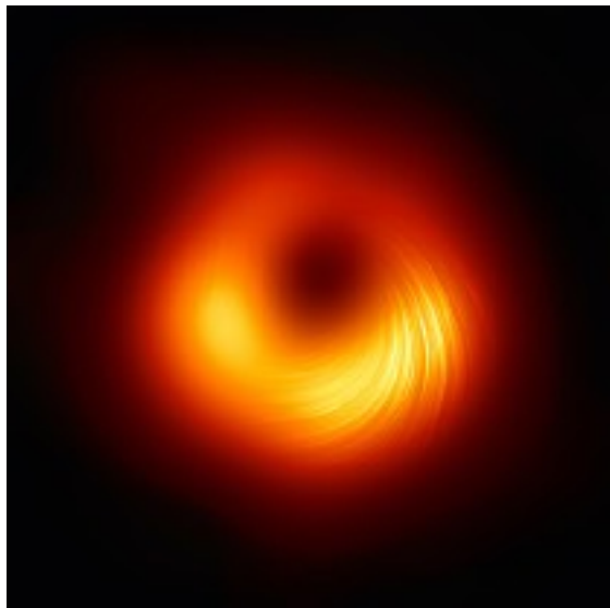
M87 (EHT 2021)
