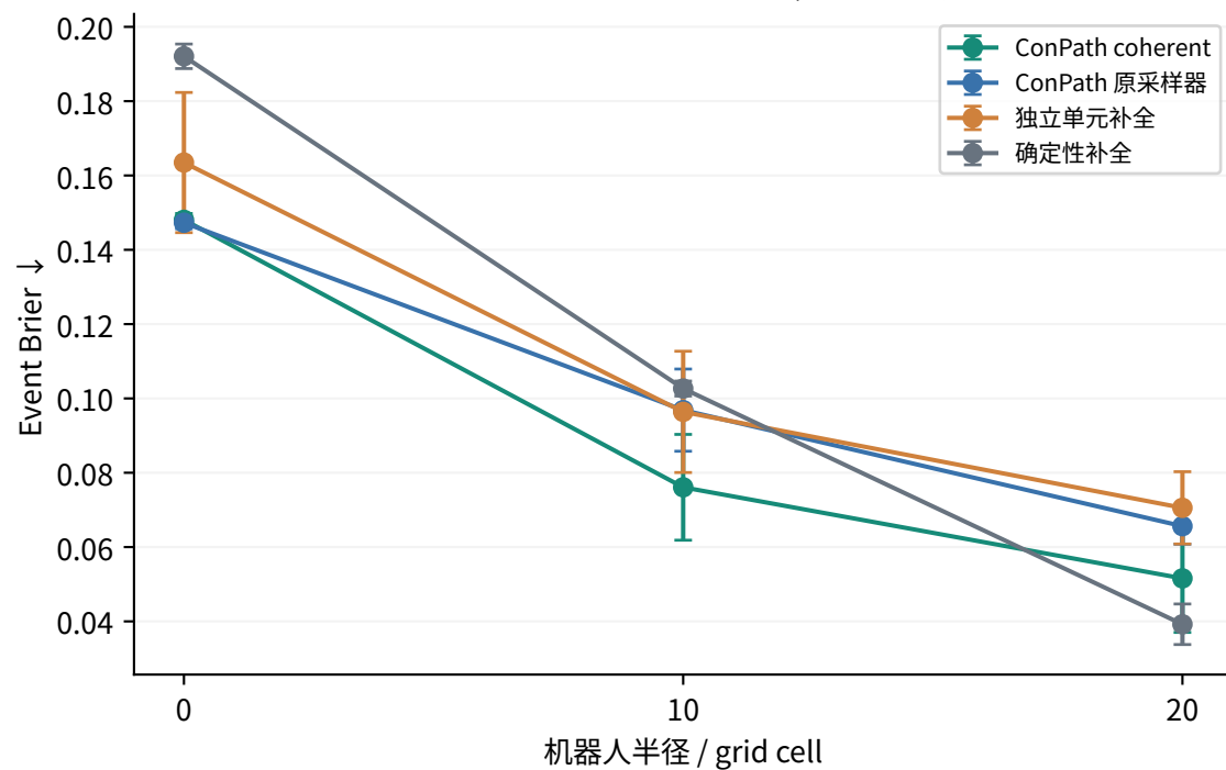
补充：coherent匹配比较，两个种子
