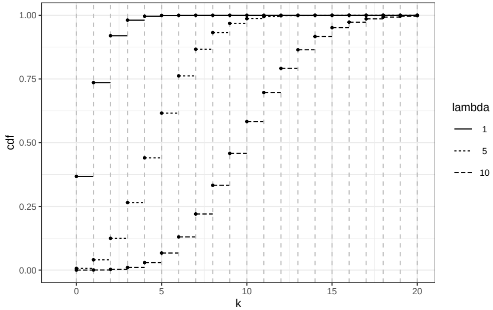
FIGURE 2.1 : Fonctions de répartition de lois de Poisson pour différents paramètres. On observe que, apparemment, \mu \leq \nu \Rightarrow F_\mu \geq F_\nu . Comment établiriez-vous cette propriété de domination ?
