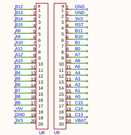
扩展引脚
