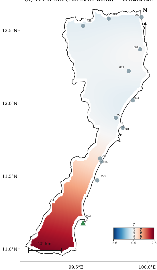
(d) TFPW-MK (Yue et al. 2002) — Z Statistic
