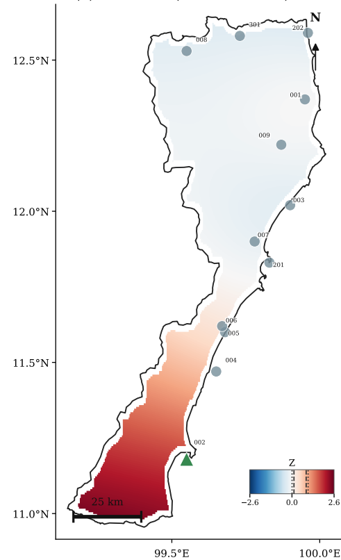
(d) TFPW-MK (Yue et al. 2002) — Z
