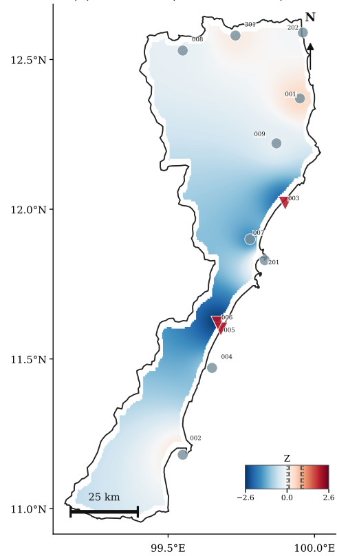
(d) TFPW-MK (Yue et al. 2002) — Z
