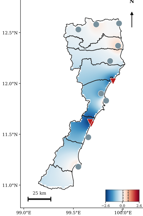
(d) TFPW-MK (Yue et al. 2002) — Z Statistic
