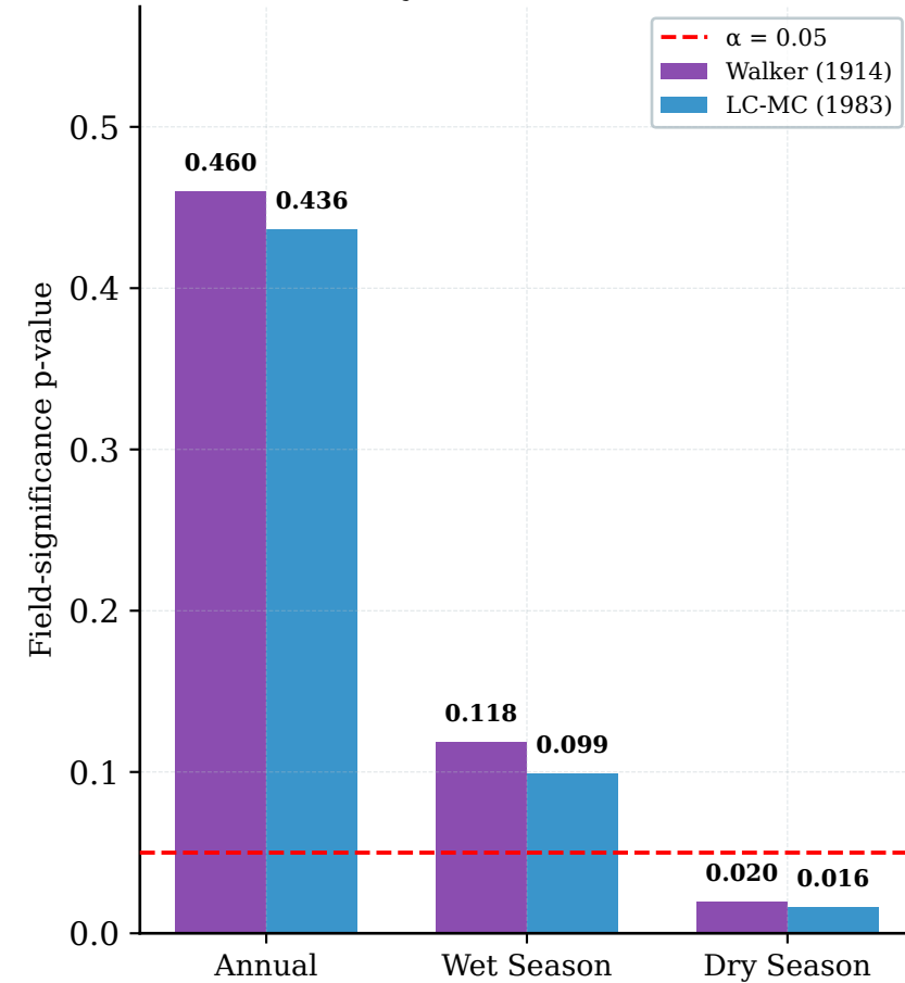
(d) Field Significance Walker & Livezey-Chen MC
