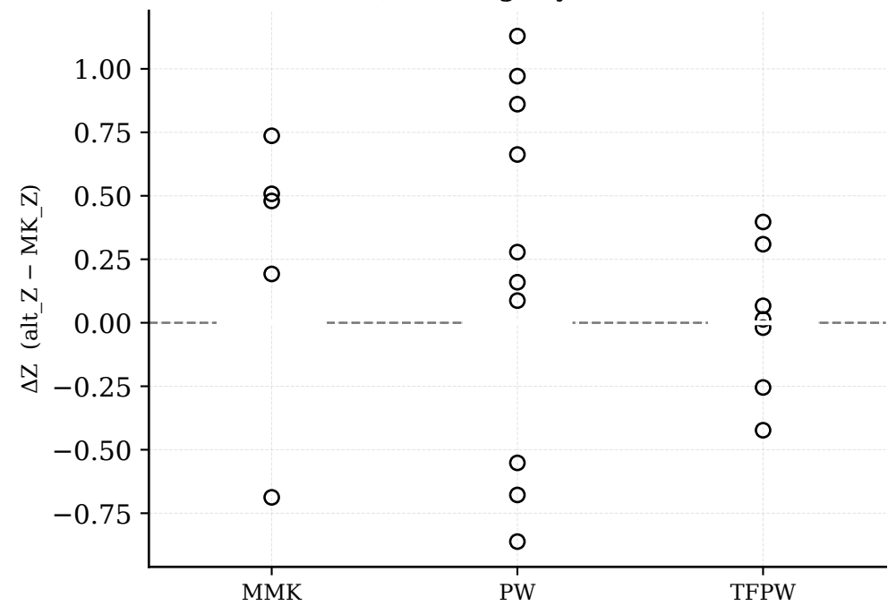
(d) \Delta Z Range by Method
