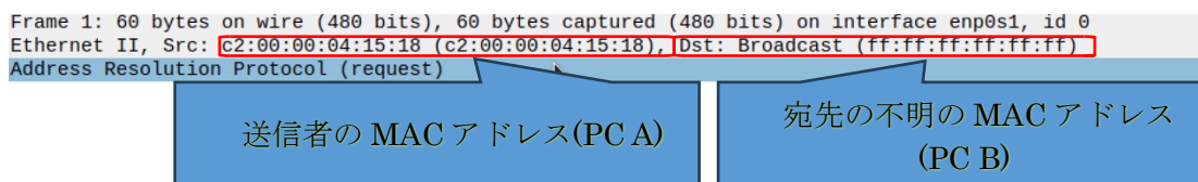
図7 フレーム 1 の詳細(request)
