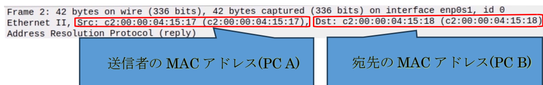
図8 フレーム 2 の詳細(reply)
