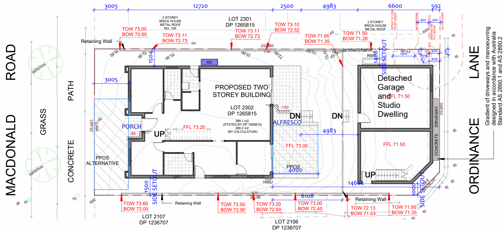
1 CC - SITE PLAN 1 : 200
