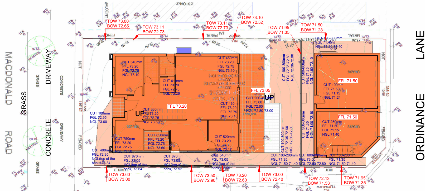
2 CUT AND FILL 1 : 200
