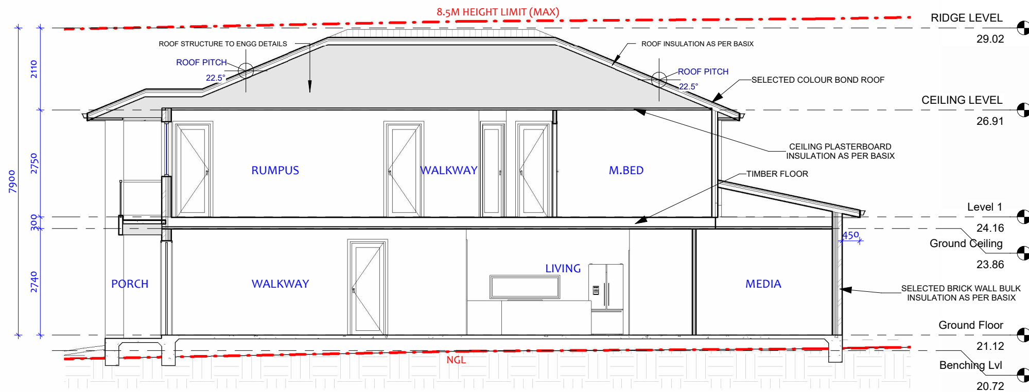
2 LONGITUDINAL SECTION 1 : 100
