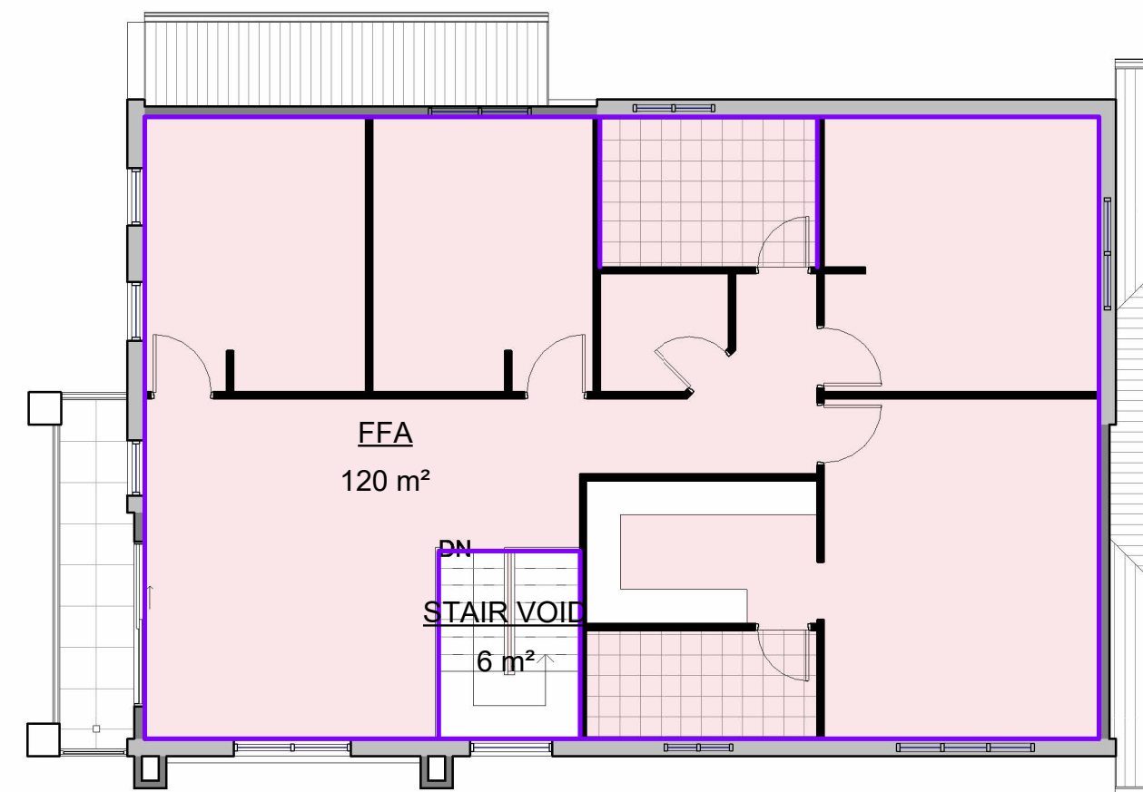
2 Level 1 1 : 100
