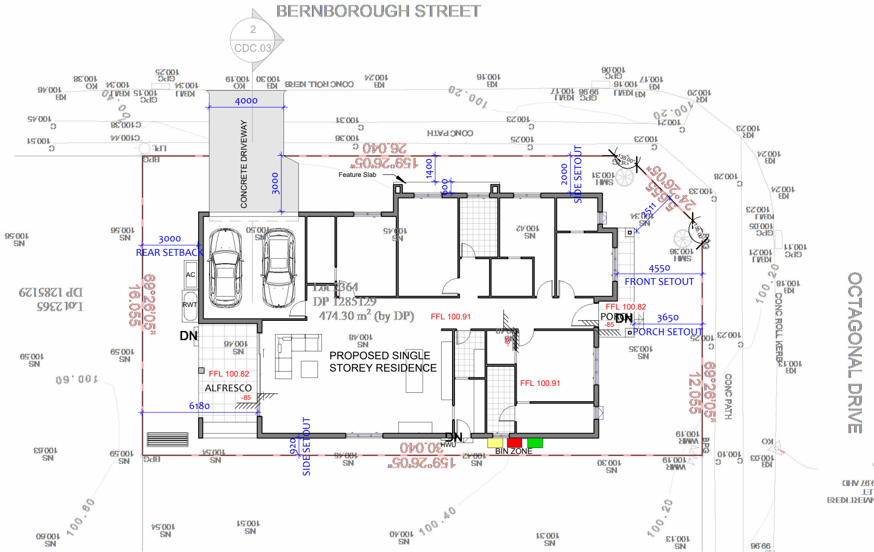
1 CDC - SITE PLAN 1 : 200
