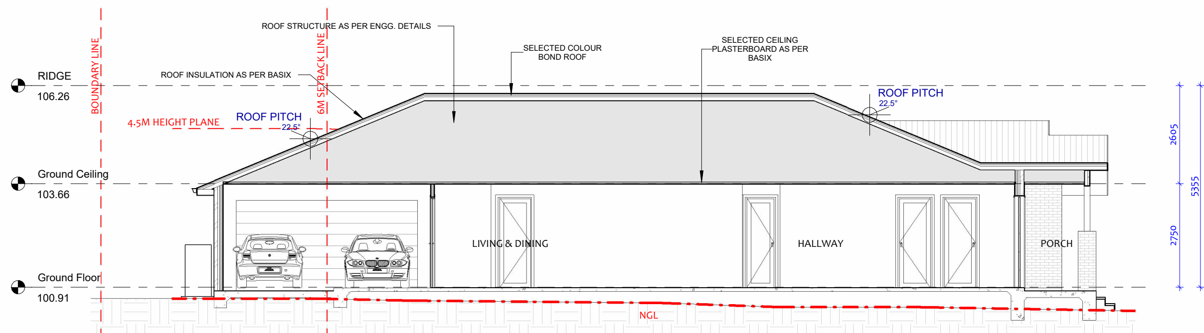
1 LONGITUDINAL SECTION 1 : 100
