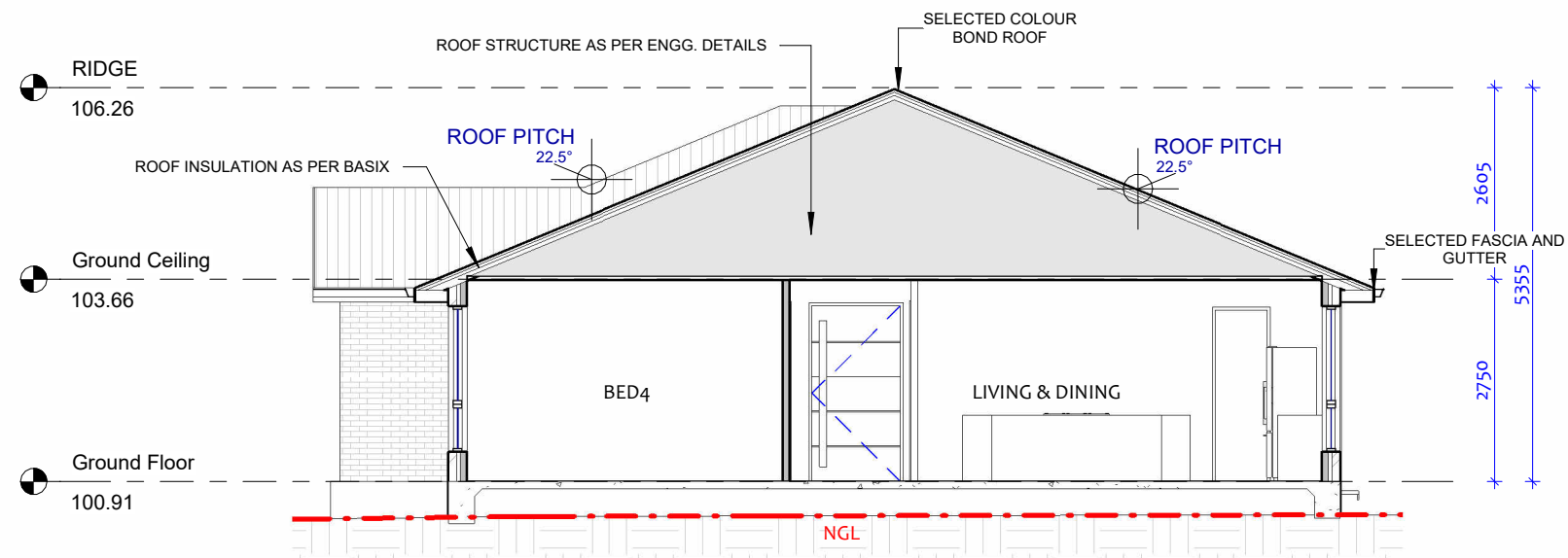
2 CROSS SECTION 1 : 100
