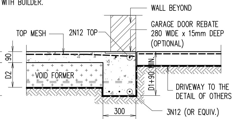
GARAGE EDGE BEAM – 'EB3'
