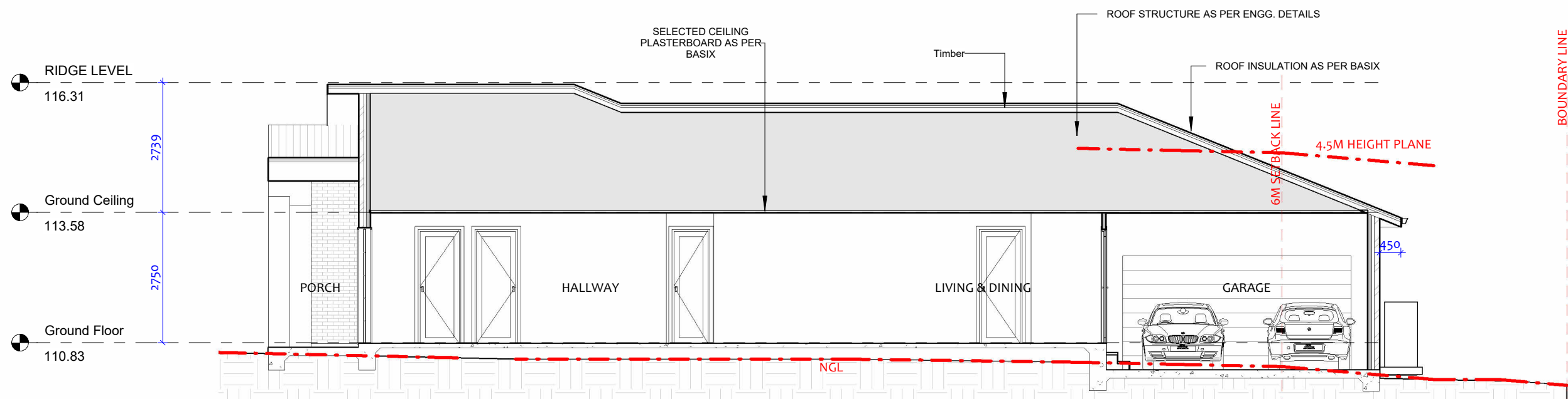
1 LONGITUDINAL SECTION 1 : 100
