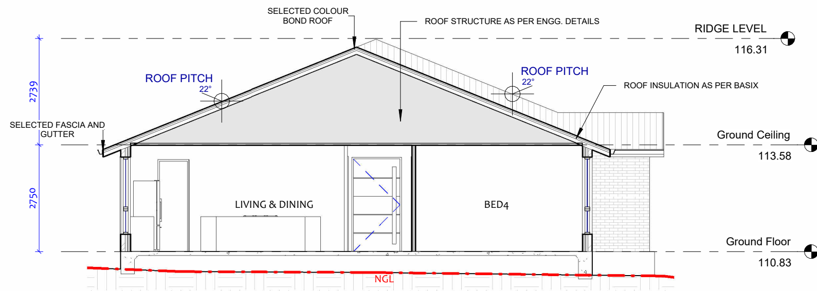
2 CROSS SECTION 1 : 100
