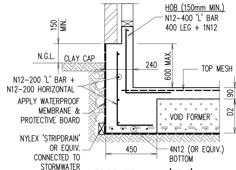
EDGE BEAM - 'EB5'
