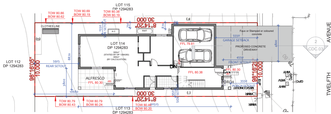
1 CDC - SITE PLAN 1 : 200
