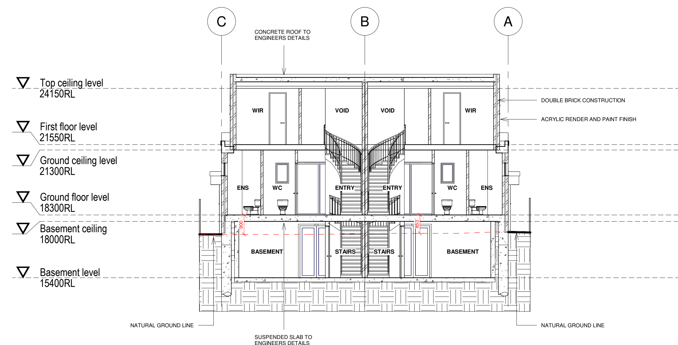
2 Section A-A 1:100
