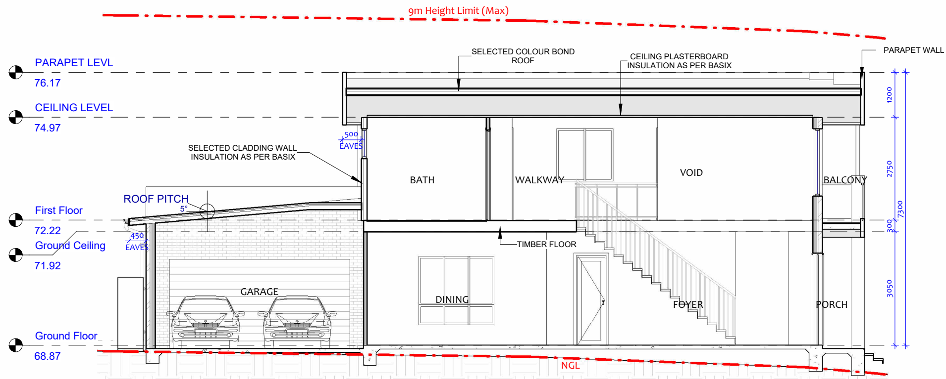
2 LONGITUDINAL SECTION 1 : 100
