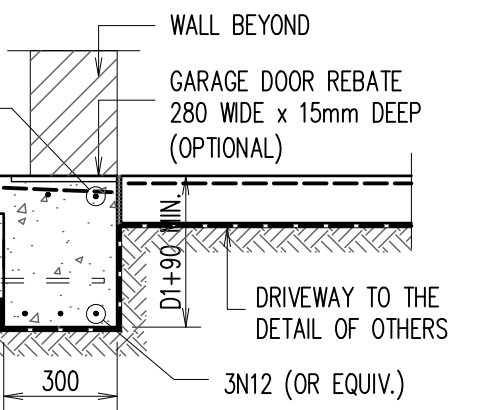
GARAGE EDGE BEAM – 'EB3'
